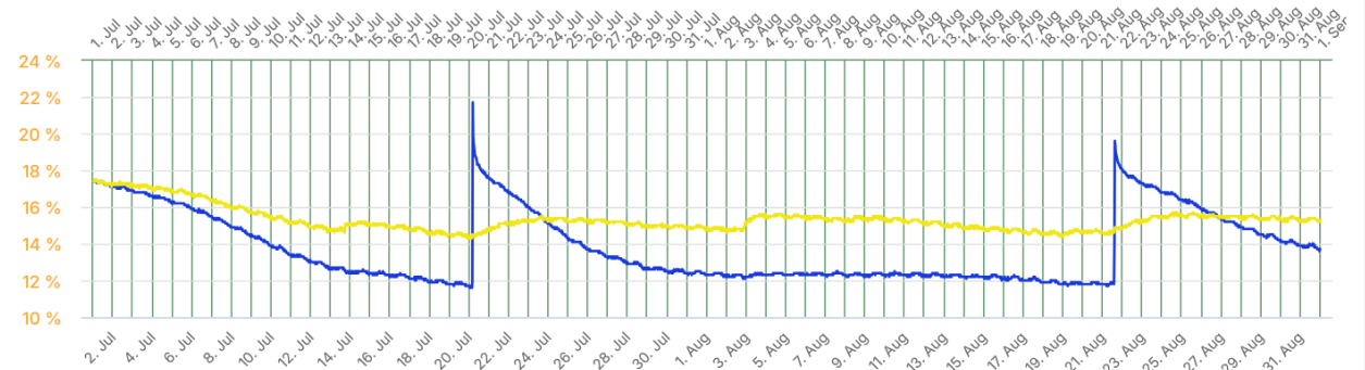
Vlažnost tal (%) 01/07/2024 - 31/08/2024
